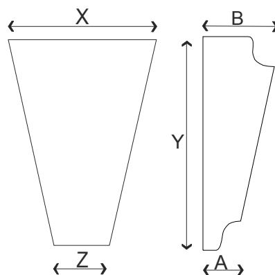
ZWORNIKI
